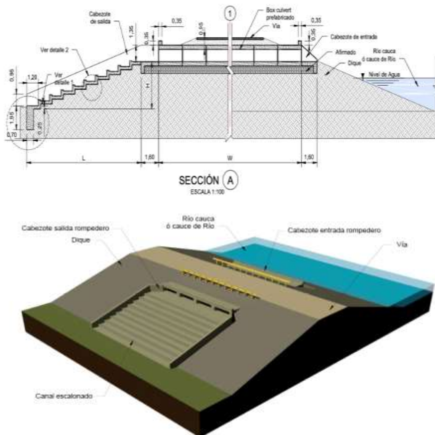
Ilustración 7 Detalle de estructuras de derivación
