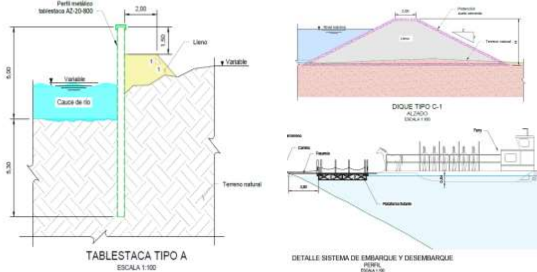
Ilustración 8 Detalle de obras de protección de los cascos urbanos
