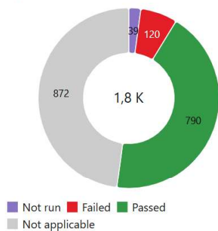
Aceptacion_SEG_Entrega1 - Chart
