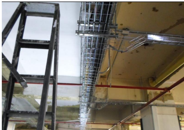
Instalación de infraestructura nueva (Bandejas portacable, tubería EMT y accesorios)
