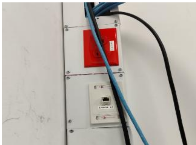
Instalación de puntos de red y toma en sala de sonido
