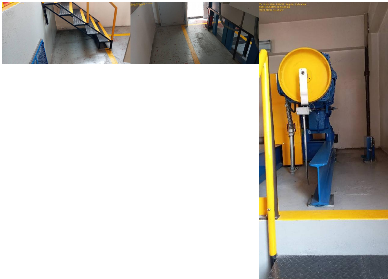
Cuarto de Maquinas - Después
