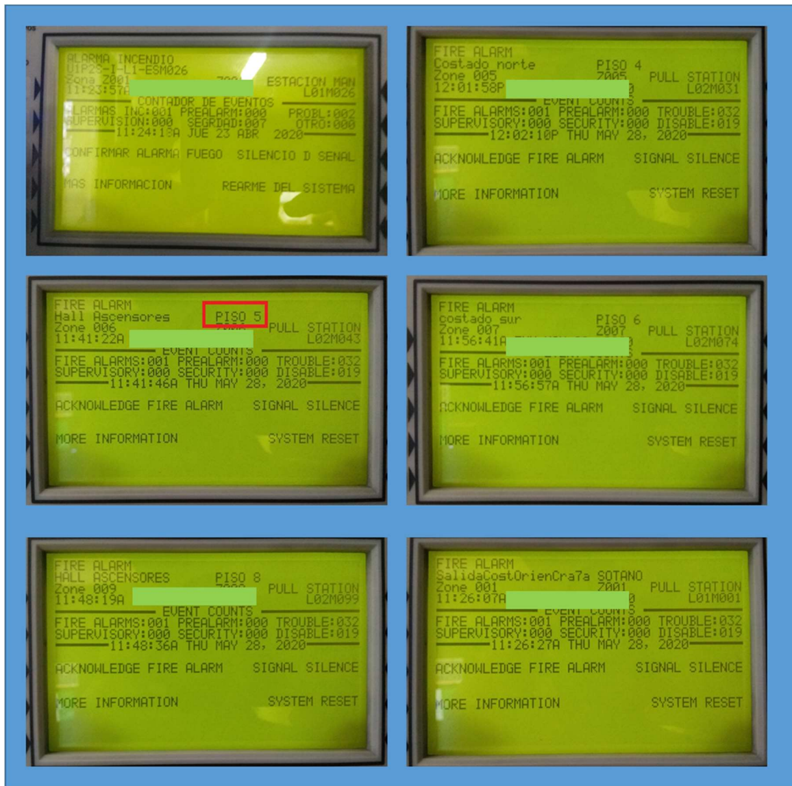
FIGURA 2. ACTIVACION EN PÁNEL DE INCENDIO
