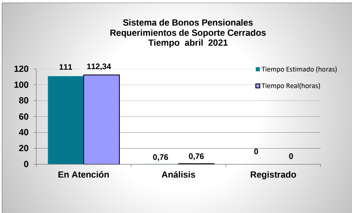
Gráfica 35 – Requerimientos de Soporte Cerrados Tiempo Estimado Vs. Tiempo Real por Estado
