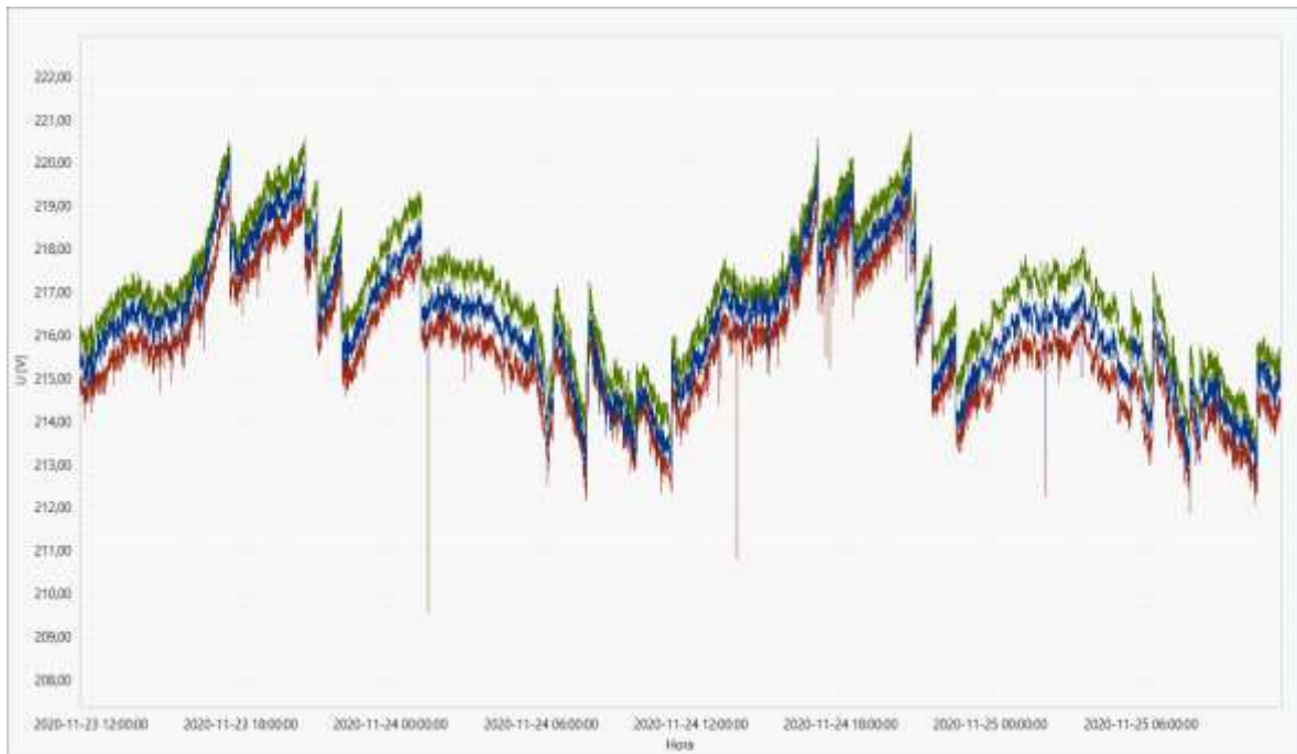
Ilustración 11 Perfil Tensión (V)
