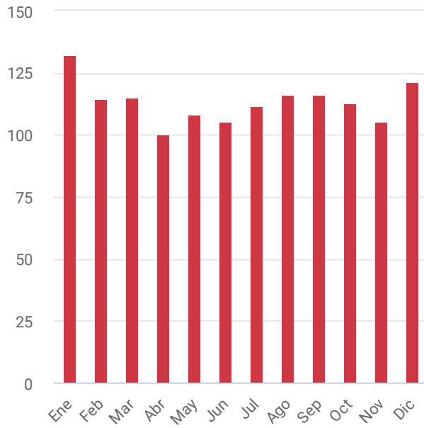
Figura 5.1: Producción fotovoltaica específica
