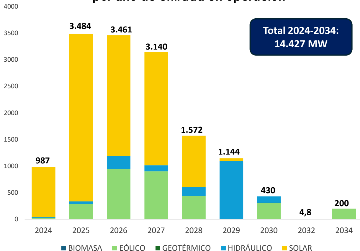
Capacidad (MW) de proyectos por año de entrada en operación
